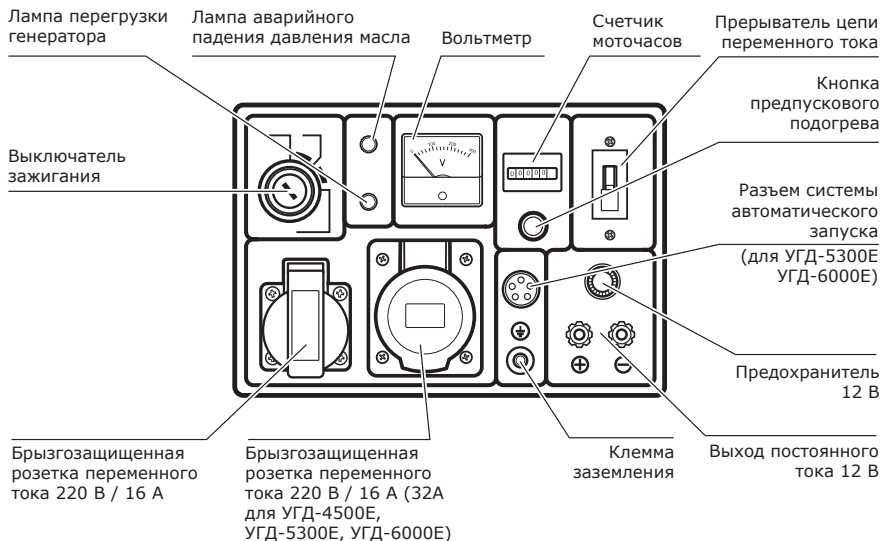
Рис. 2. Схема панели управления генераторов УГД-3000Е, УГД-4500Е, УГД-5300Е, УГД-6000Е.
