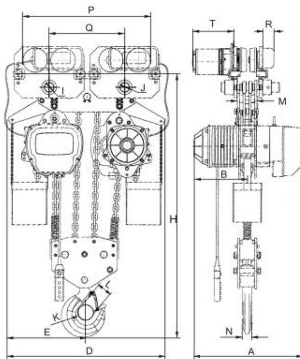
Рисунок 3. Габаритные размеры ННВД-Т 10т
