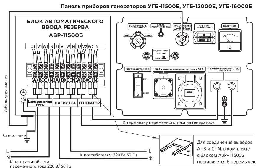
Рис. 21. Рекомендуемая схема подключения резерва АВР-11500Б (3 фазы)
