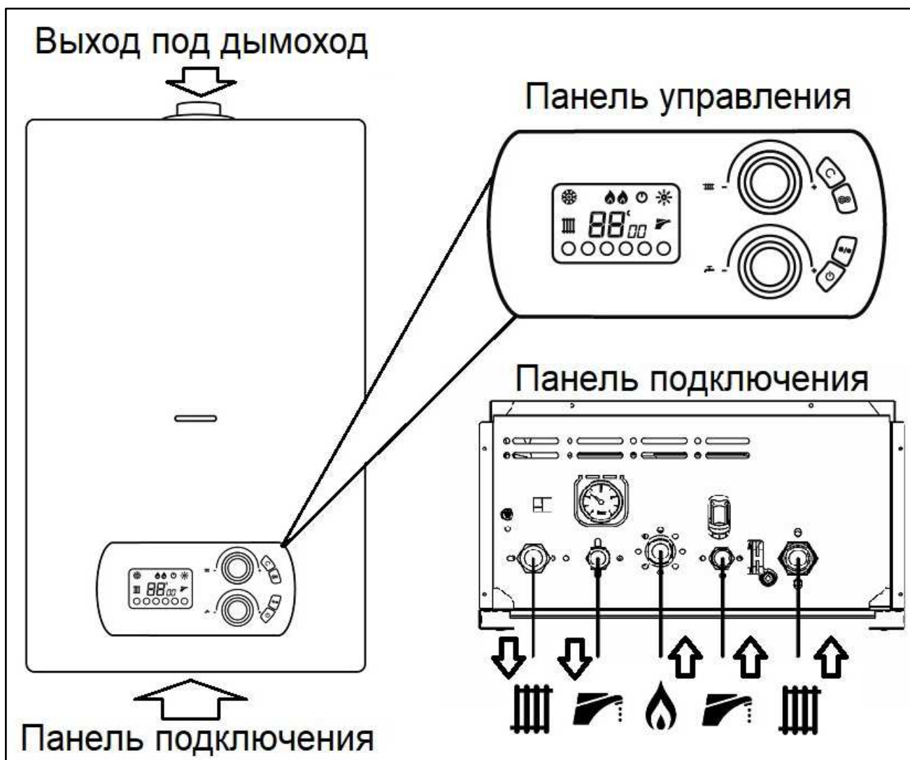
Рис. 1. Общий вид газового котла
