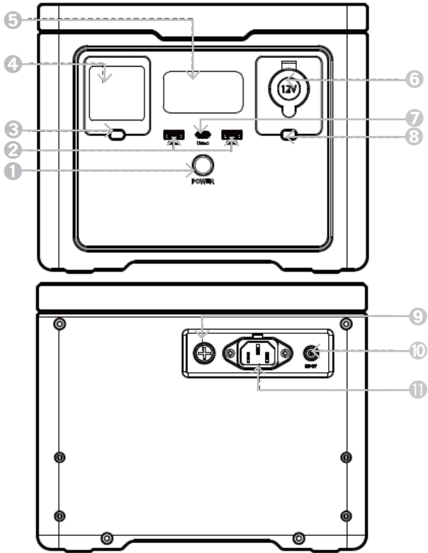
Рисунок 1.5. Устройство инструмента
