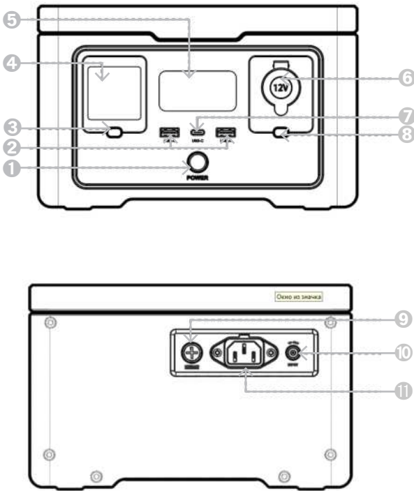
Рисунок 1.5. Устройство инструмента
