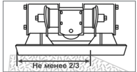
Рис. 15 Расположение виброплиты на краю обрабатываемой поверхности
