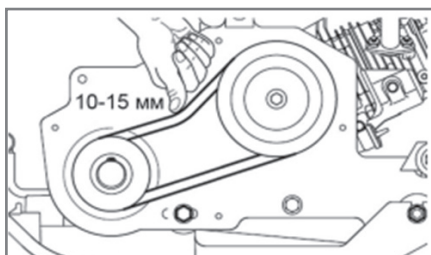
Рис. 22 Проверка натяжения ремней
