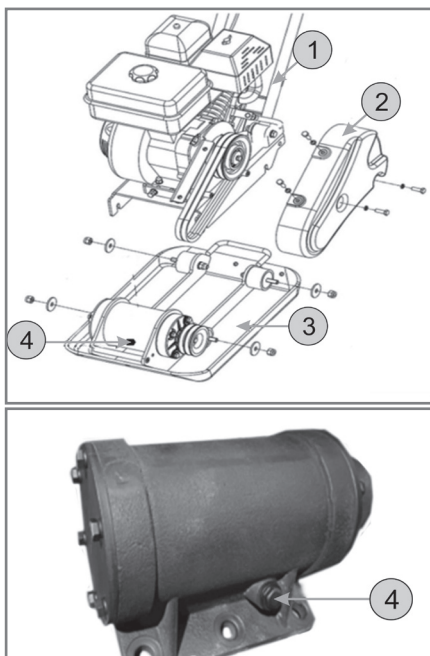
Рис. 25 Замена масла в виброузле 1 - Рама с установленным двигателем и рукоятками, 2 - Кожух защитный ремней, 3 - Плита рабочая, 4 - Пробка слива и заправки масла.
