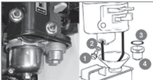
Рис. 20 Обслуживание фильтра отстойника
