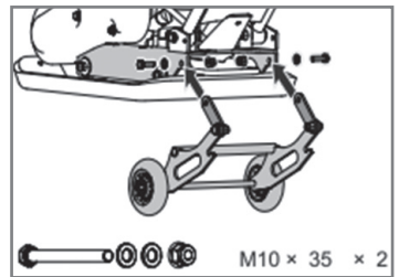
Рис. 4 Установка транспортировочной тележки
