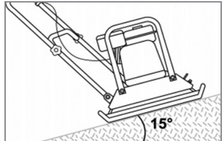
Рис. 16 Максимальный угол наклона виброплиты
