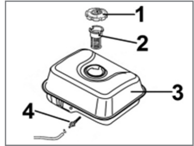
Рис. 19 Расположение топливных фильтров
