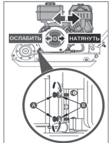
Рис. 24 Регулировка натяжения ремней
