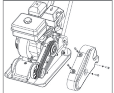
Рис. 23 Замена ремней
