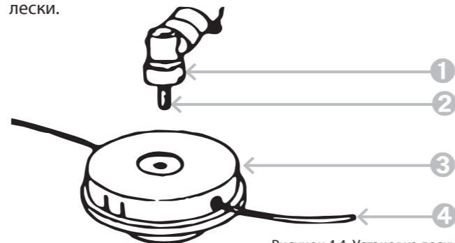
Рисунок 4.4. Установка лески
