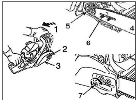
Рис. 2 Установка шины
