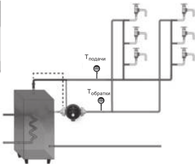
4-сүр. Температуранын эки билдиргичи менен COMFORT соркысмасы ЫСК тутумунда
