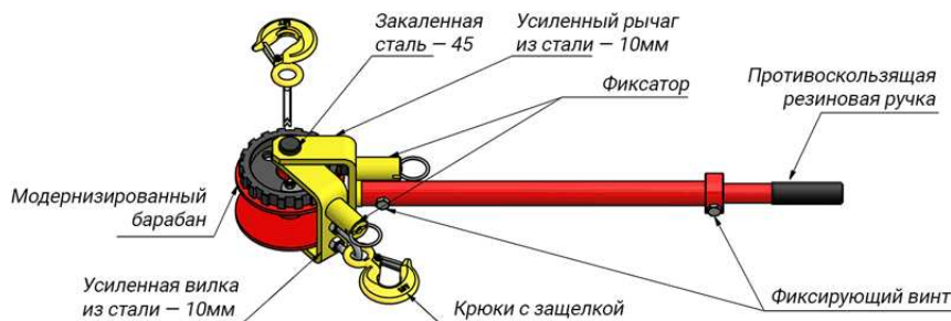
Рисунок 1. Устройство лебедки ручного рычажного модели ЛР.
