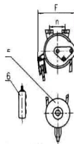
Рис. 10 - Электрическая таль CD1 10 т-20т, 6 - 36 м с жестким креплением
