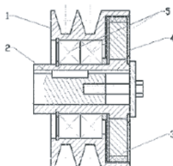
Рис. 2 Устройство муфты сцепления
