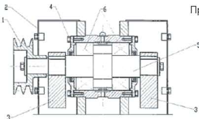
Рис. 1 Устройство дебаланса 1 – шкив, 2 – крышка дебаланса, 3 – дебаланс, 4 – крышка, 5 – вал дебаланса, 6 – подшипник 3610
