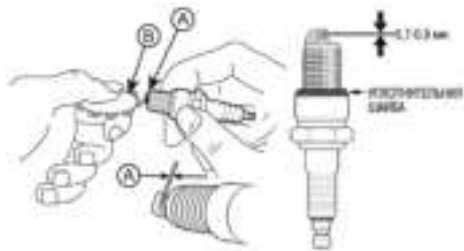
Рис. 42 Проверка межэлектродного зазора А- зазор В- щуп
