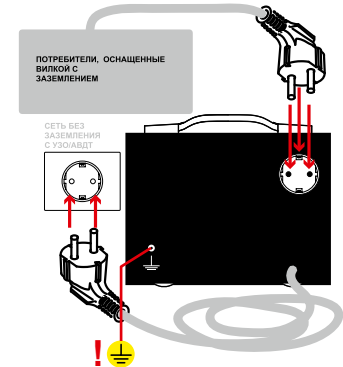
Схема подключения стабилизатора в сеть без заземляющего провода, с УЗО
