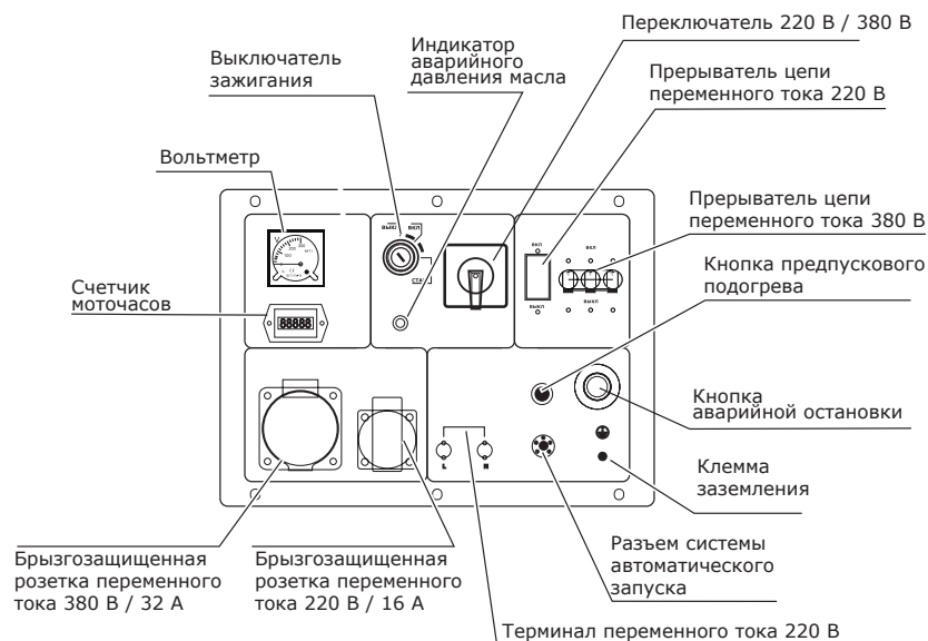
Схема панели управления генераторов УГД-11500ЕТ PROFF, УГД-15000ЕТ PROFF.
