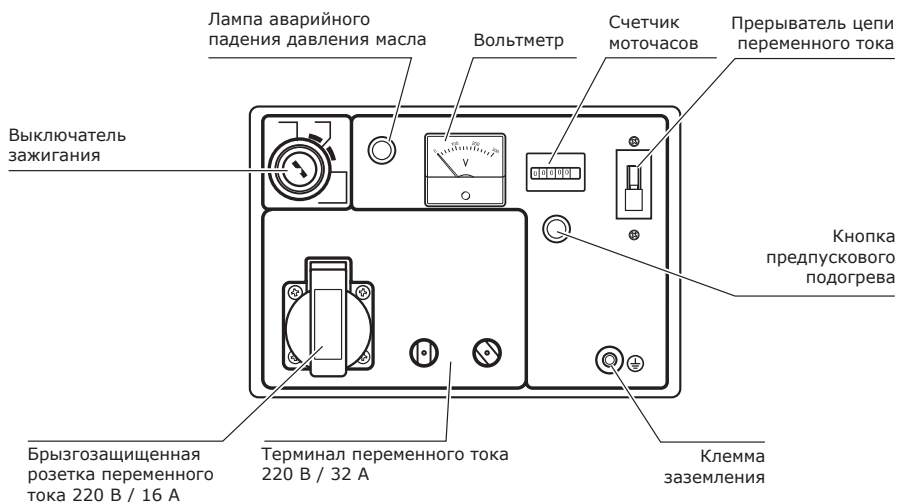
Схема панели управления генераторов УГД-9500E PROFF, УГД-11000E PROFF.
