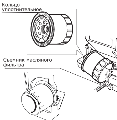
Рис. 24. Замена масляного фильтра.
