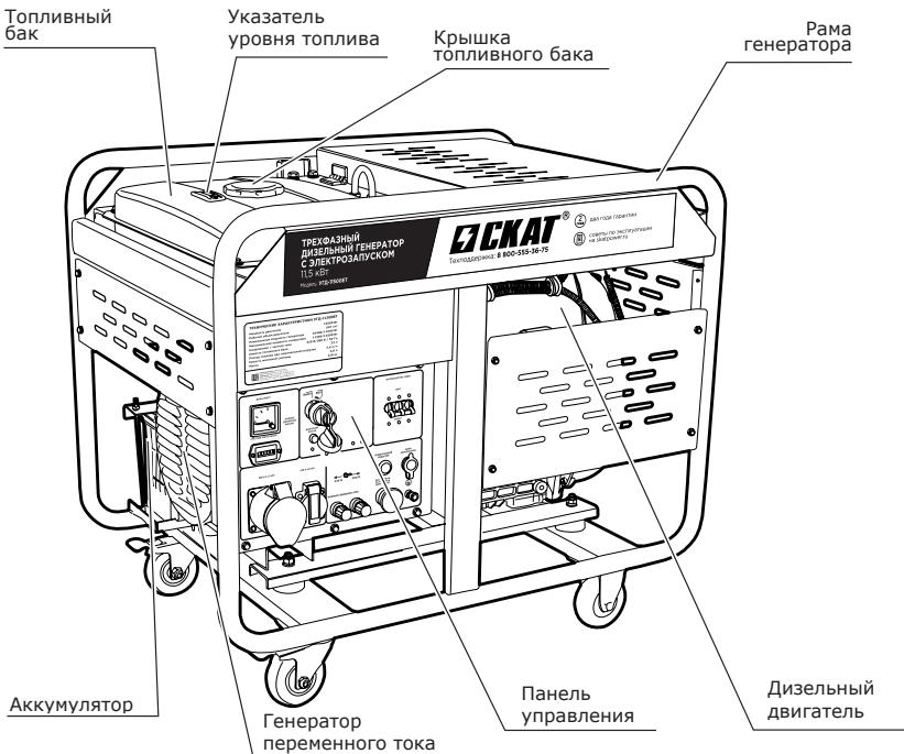
Рис. 3. Общий вид генераторов УГД-11500Е PROFF, УГД-11500ЕТ PROFF, УГД-15000Е PROFF, УГД-15000ЕТ PROFF.
