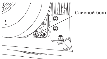
Рис. 23. Сливной болт.
