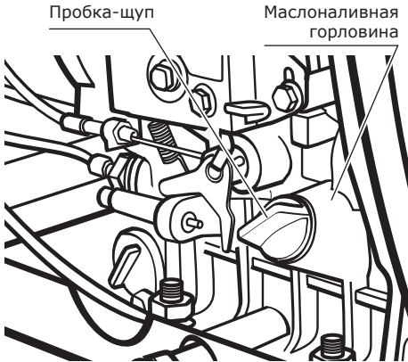
Рис. 7. Заполнение масляного картера и контроль уровня масла.
