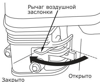
Рис. 15. Рычаг привода воздушной заслонки
