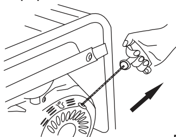
Ручка стартера
