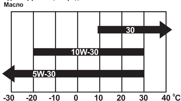
Рис.6 Диаграмма соответствия требуемой вязкости масла температуре окружающей среды
