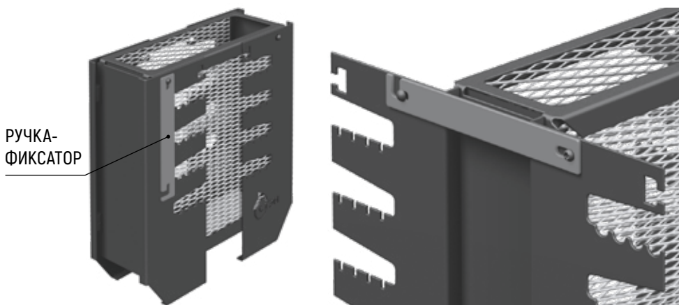
Рис.1. Сборка мангала
