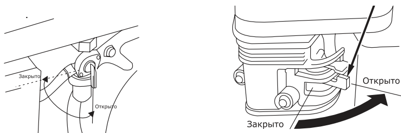
Рис. 14. Топливный кран
