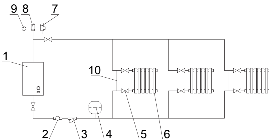
Рис. 5. Упрощённая схема подключения электродкотла в закрытую отопительную систему с циркуляционным насосом.
