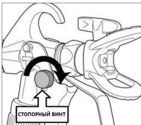
Рис. 11. Блокировка пистолета-распылителя
